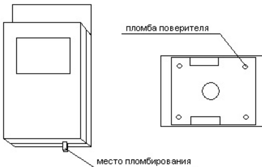
Рисунок 2 – Схема пломбировки от несанкционированного доступа, обозначение места нанесения знака поверки (TeRoss-ВУ – слева, TeRoss-ИБ – справа)
